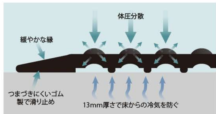
断面図と機能図
